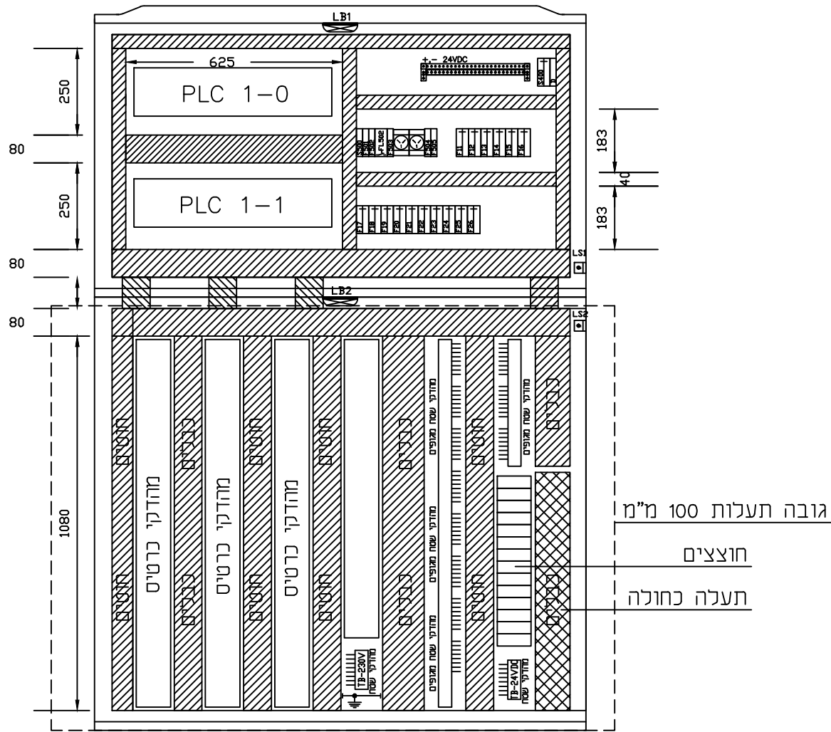
כניסות כבלים
